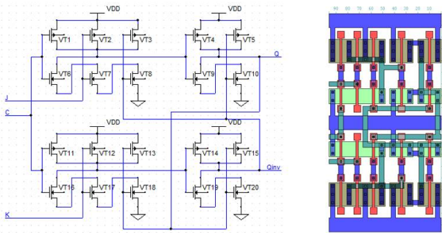
Рис. 6. Електрична схема JK-тригера на основі логічних елементів 1-HE (а) та топологія JK-тригера на основі базових матричних комірок (б).
